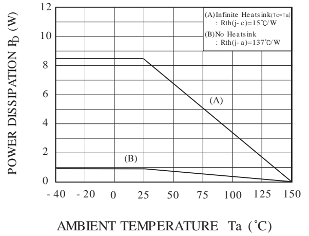
P_D - T_a ( S : SOT- 223 )
