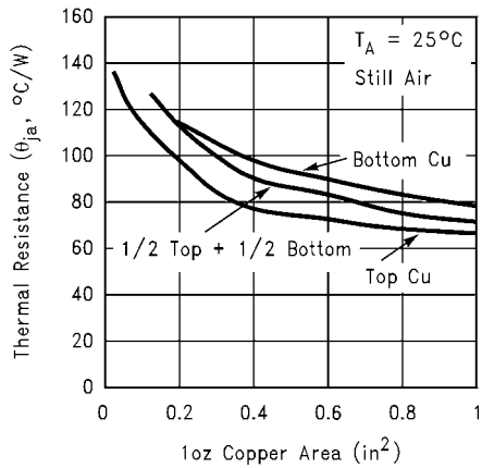
R \theta JA vs 1-oz Copper Area for SOT-223
