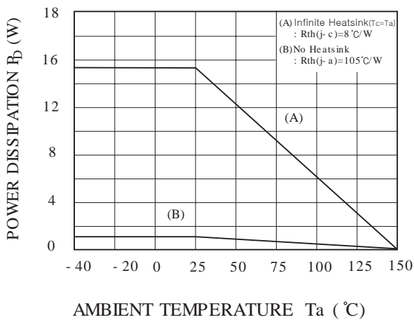
P_D - T_a ( D : D- PAK )
