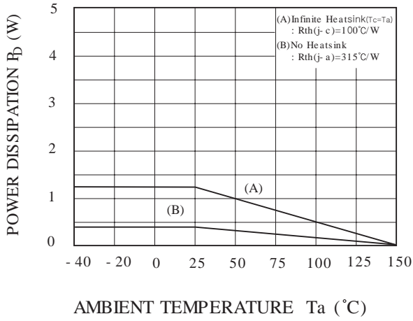
P_D - T_a ( F : SOT- 89 )
