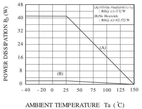
P_D - T_a ( P : TO-220 )
