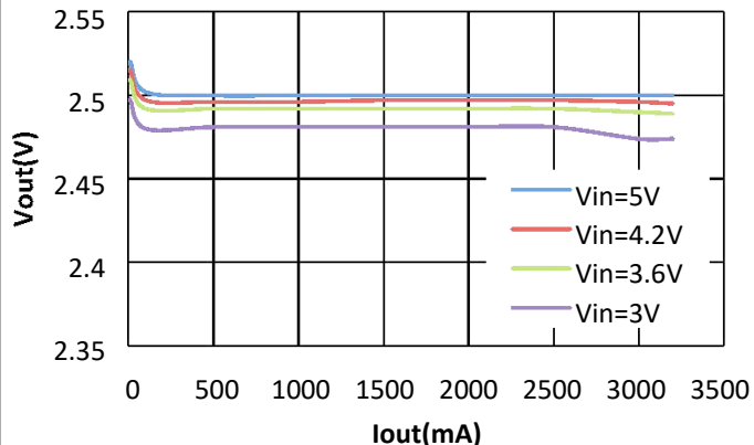
Iout vs Vout(Vout=2.5V)
