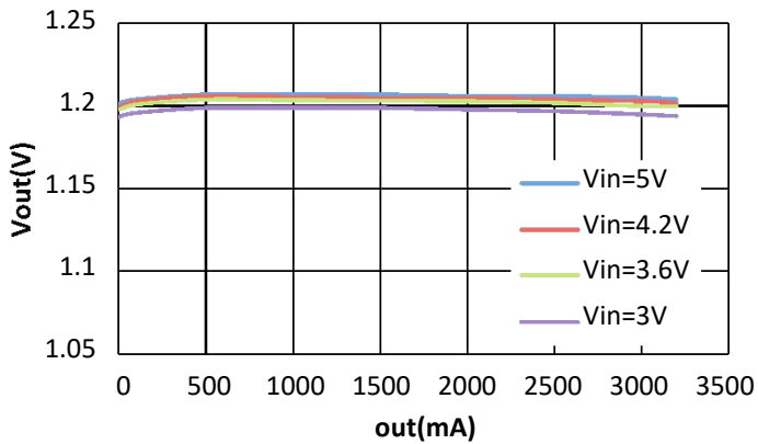
Iout vs Vout(Vout=1.2V)
