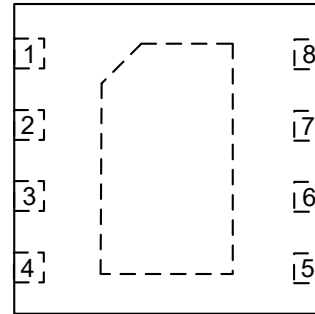
DFN3*3-8L
