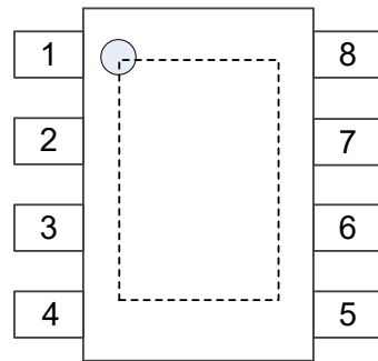
ESOP8
