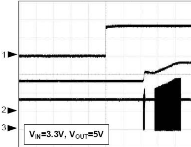
EN Goes High - Enable, No Load
