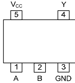
SOT-23-5/SOT-25 SOT-353/SOT-553
