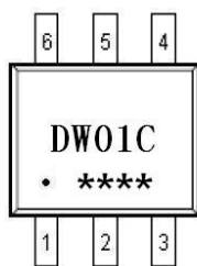
SOT23-6
