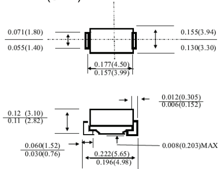
DO - 214AA(SMB)
